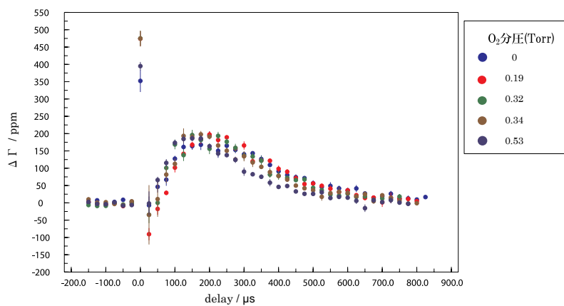
図2 異なる O_2 分圧での MnO ラジカルの吸収量の時間変化
