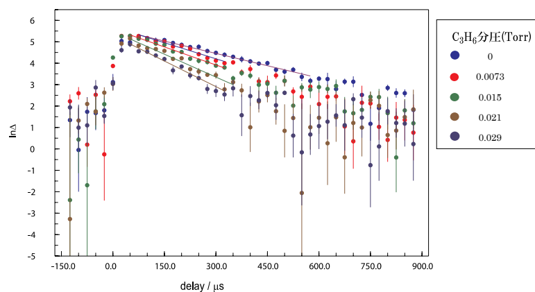
図3 異なる C_3H_6 分圧での MnO ラジカルの吸収量の時間変化
