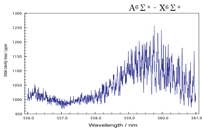
図1 MnO ラジカルの吸収スペクトル
