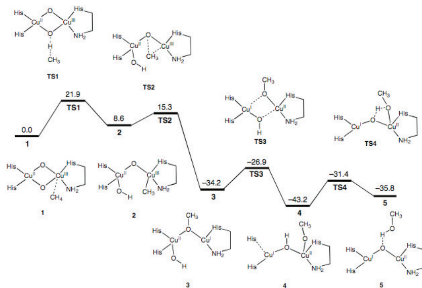
図 2. メタン-メタノール転化反応のエネルギーダイアグラム(単位は kcal/mol).
